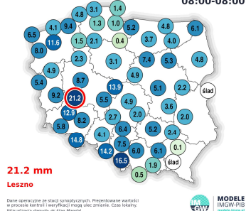
Suma opadu Piątek / Sob. 18.09.26 / 19.09.26 08:00-08:00
