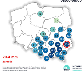
Suma opadu Niedziela / Pon. 13.09.26 / 14.09.26 08:00-08:00
