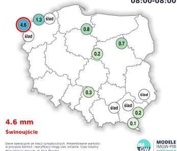
Suma opadu Czwartek / Pt. 17.09.26 / 18.09.26 08:00-08:00
