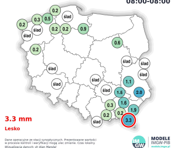
Suma opadu Poniedziałek / Wt. 14.09.26 / 15.09.26 08:00-08:00
