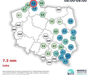
Suma opadu Sobota / Niedz. 19.09.26 / 20.09.26 08:00-08:00
