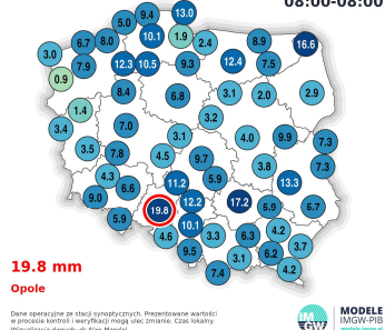
Suma opadu Niedziela / Pon. 20.09.26 / 21.09.26 08:00-08:00
