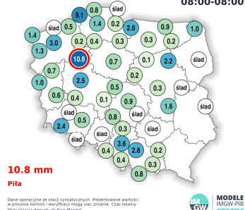
Suma opadu Wtorek / Śr. 15.09.26 / 16.09.26 08:00-08:00
