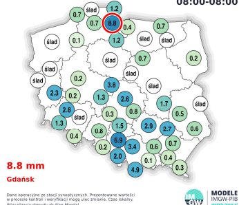
Suma opadu Środa / Czw. 16.09.26 / 17.09.26 08:00-08:00
